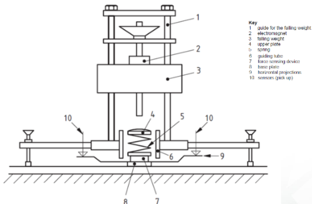
Figure 6 : Appareil de l'Athlète Artificiel – Dispositif de Déformation Verticale
